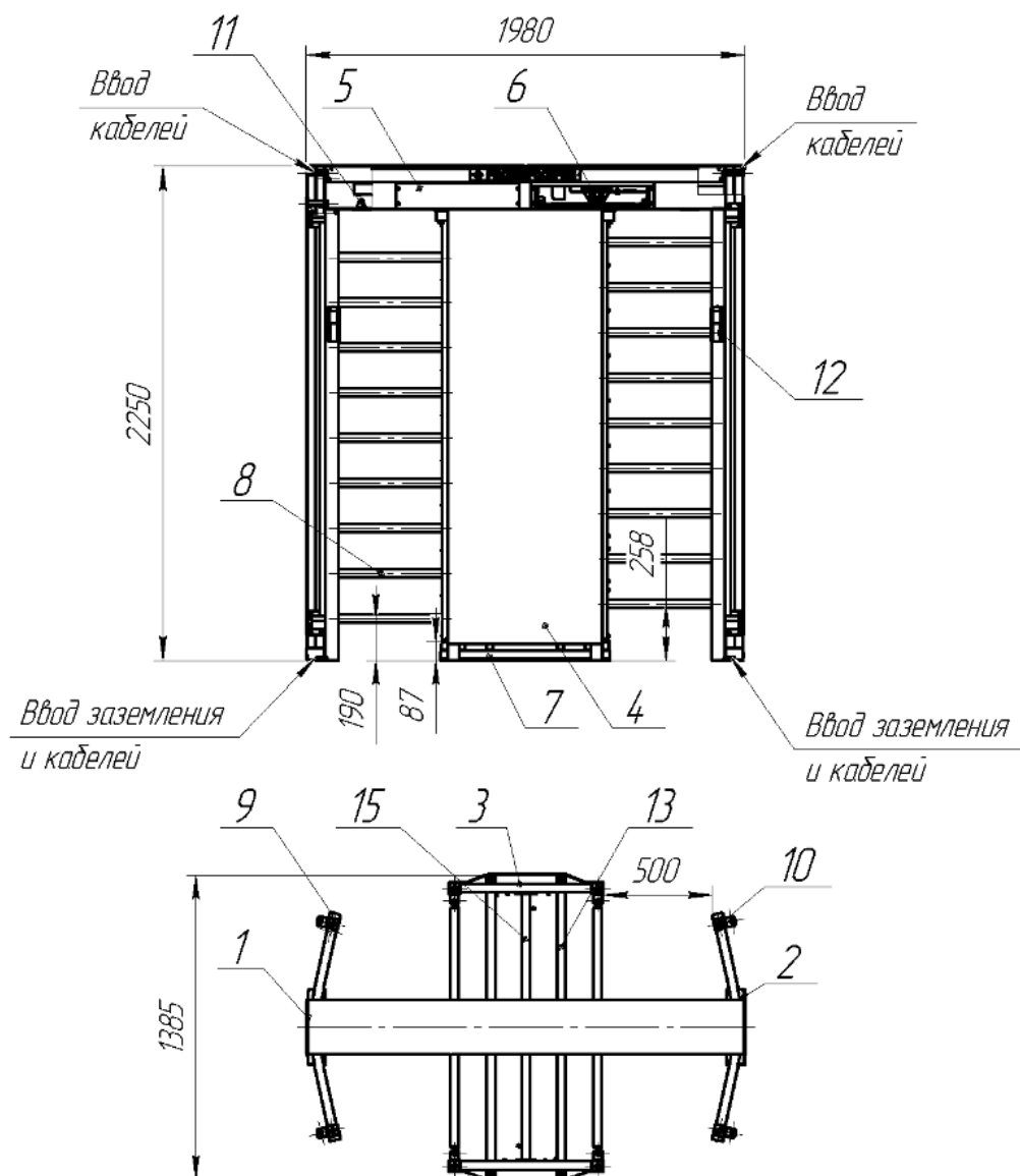
Габаритные размеры турникета «Ростов-Дон ПР2/4М-У-П»
